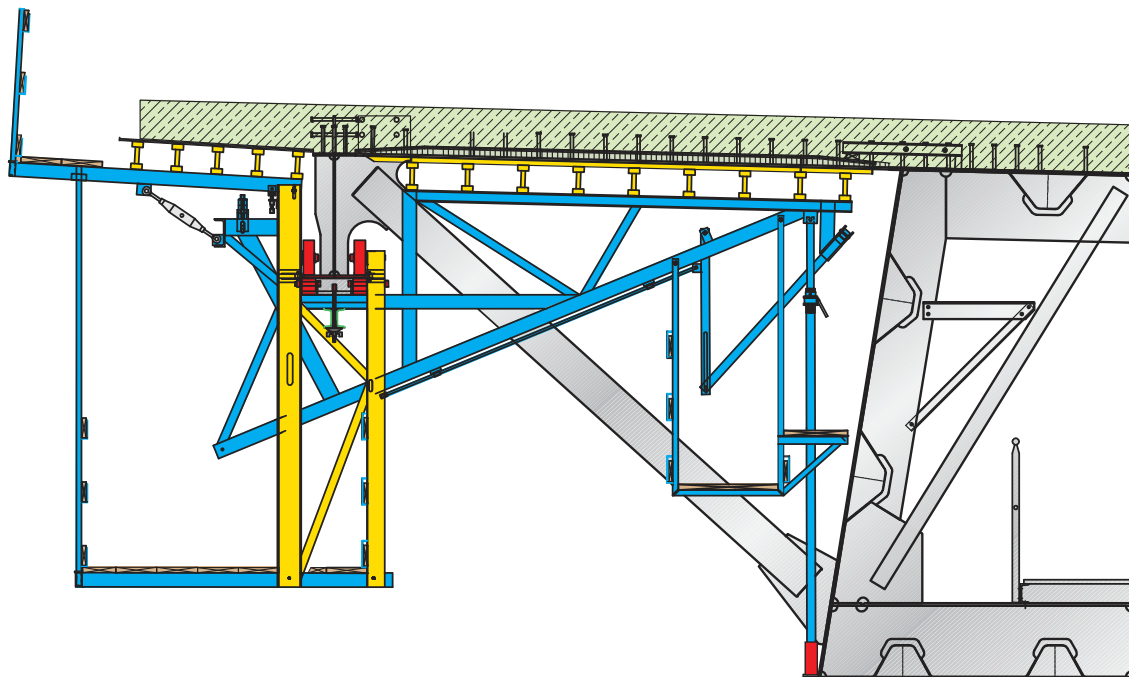
eingeschalt , Betonierzustand
