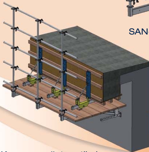
Kappengerüst vertikal
