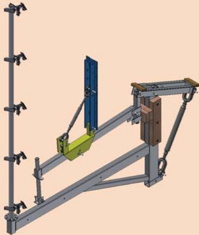
SAN-Riegel horizontal
