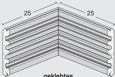
geklebtes Eckelement
