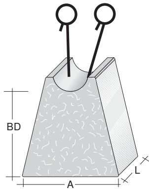
für mittelschwere Bewehrung
